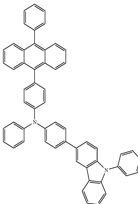
PCBAPA
