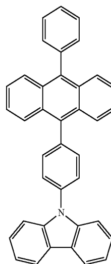
CzPA
